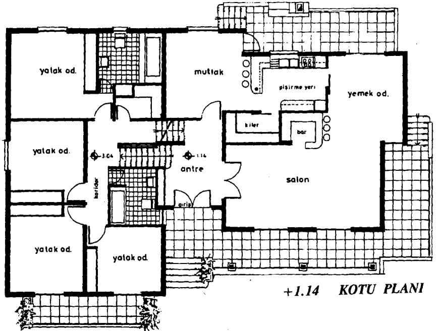
Bir Konut Tasarımının Plan ve perspektif çizimleri
