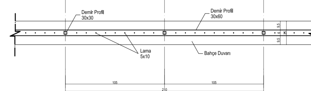
BAHÇE DUVARI PLAN Ölçek: 1/20
