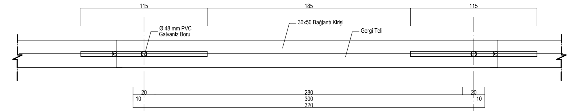
TELLEME PLAN Ölçek: 1/20
