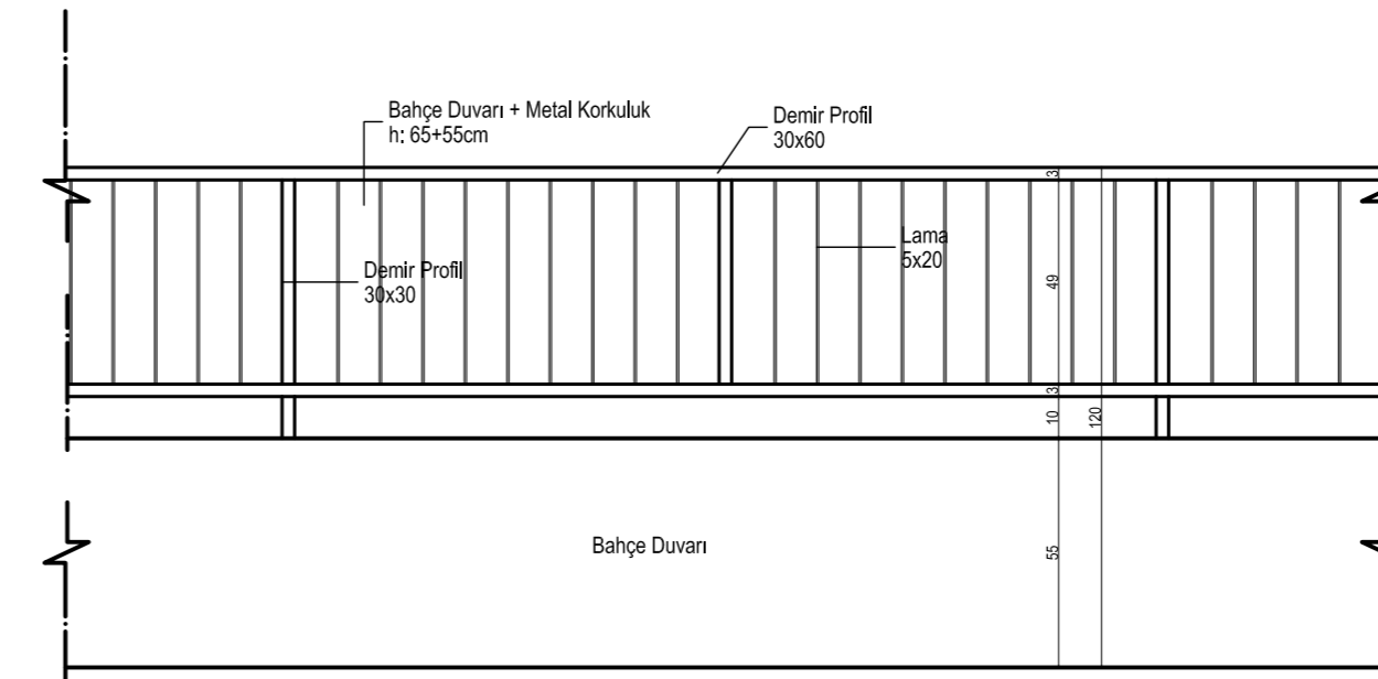
BAHÇE DUVARI ÖN GÖRÜNÜŞÜ Ölçek: 1/20
