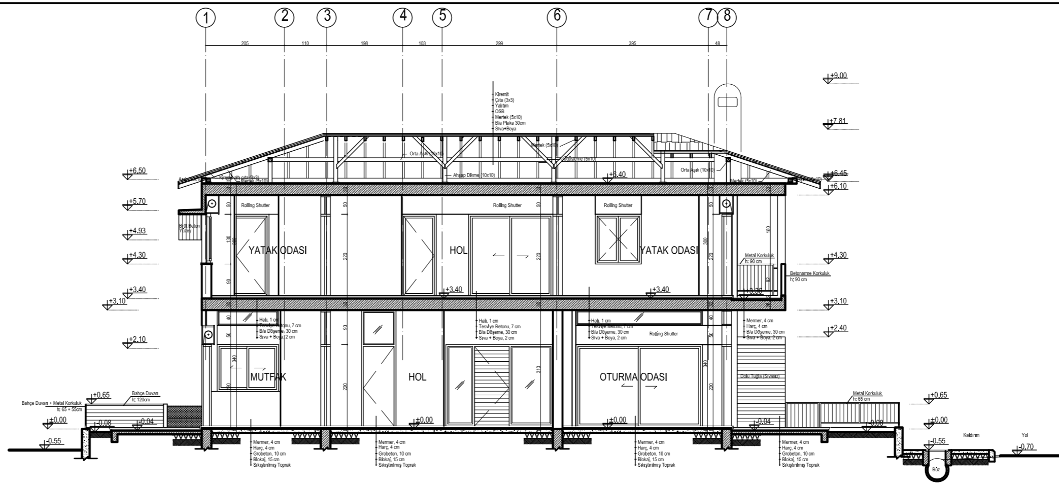
B-B KESİTİ Ölçek: 1/100
