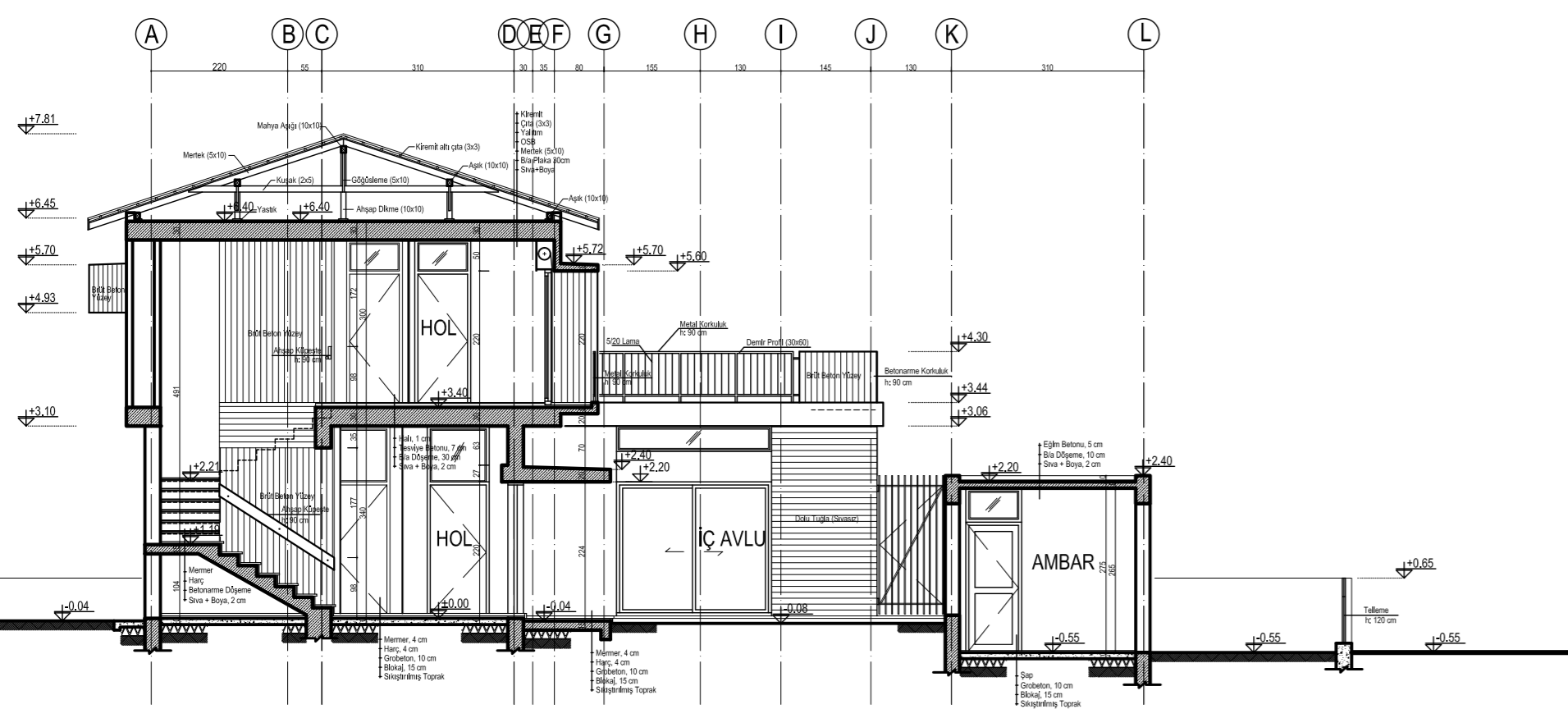
A-A KESİTİ Ölçek: 1/100
