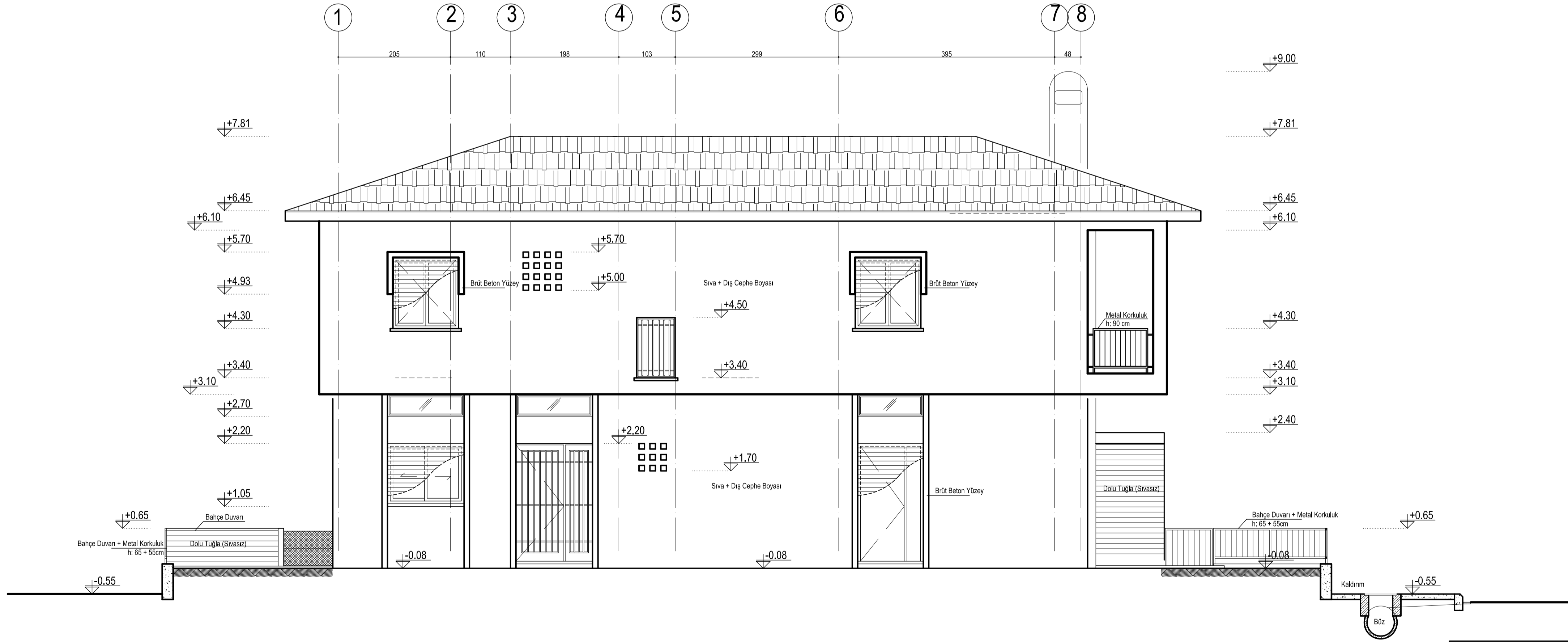
GÜNEY CEPHESİ ÖLÇEK:1/50
