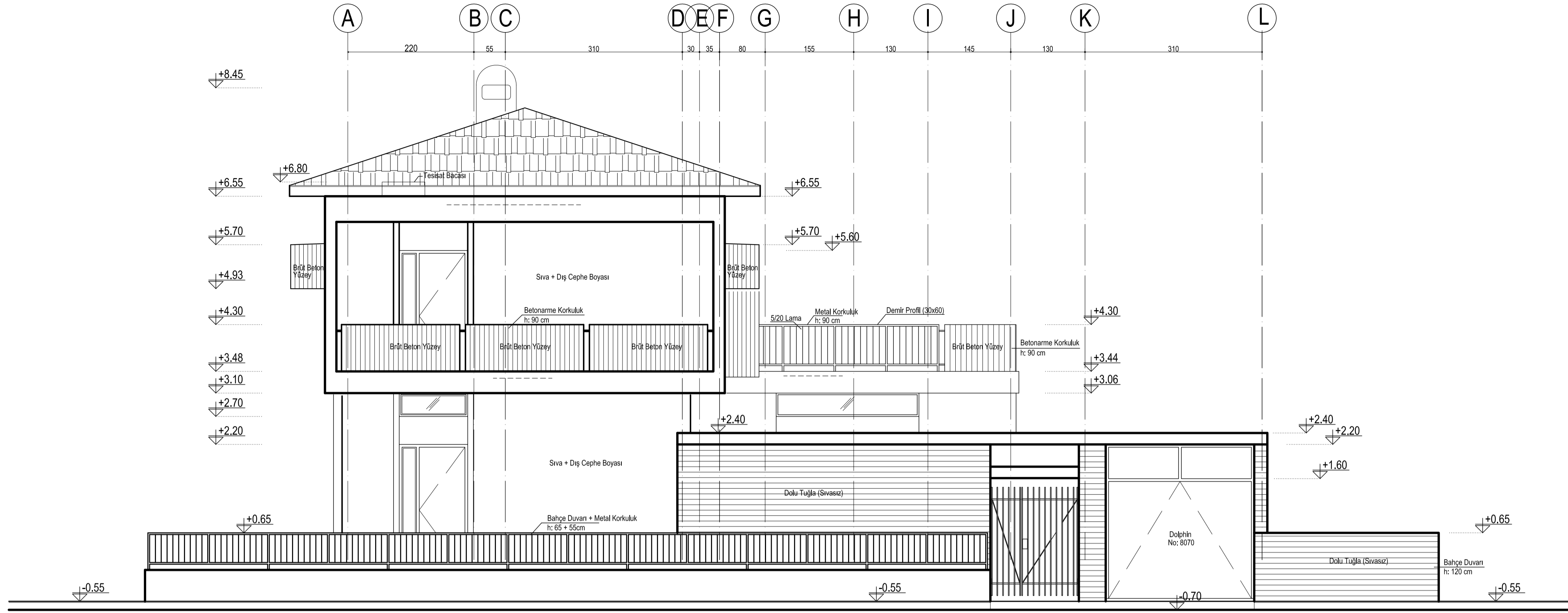
KUZEY CEPHESİ ÖLÇEK:1/50
